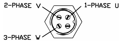
A 向视图 2:1
